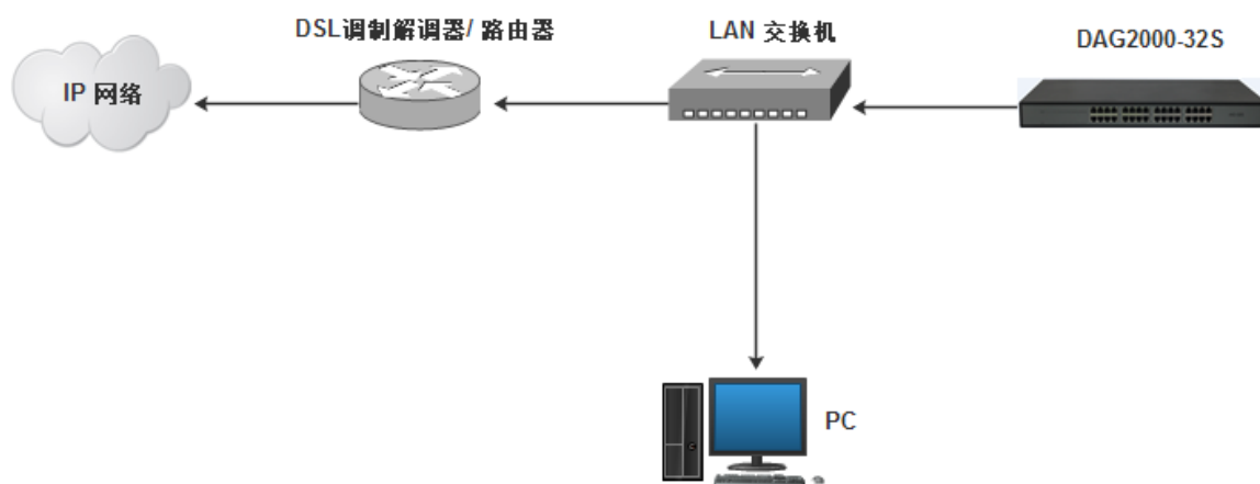
4.1-1 典型网络拓扑连接图
