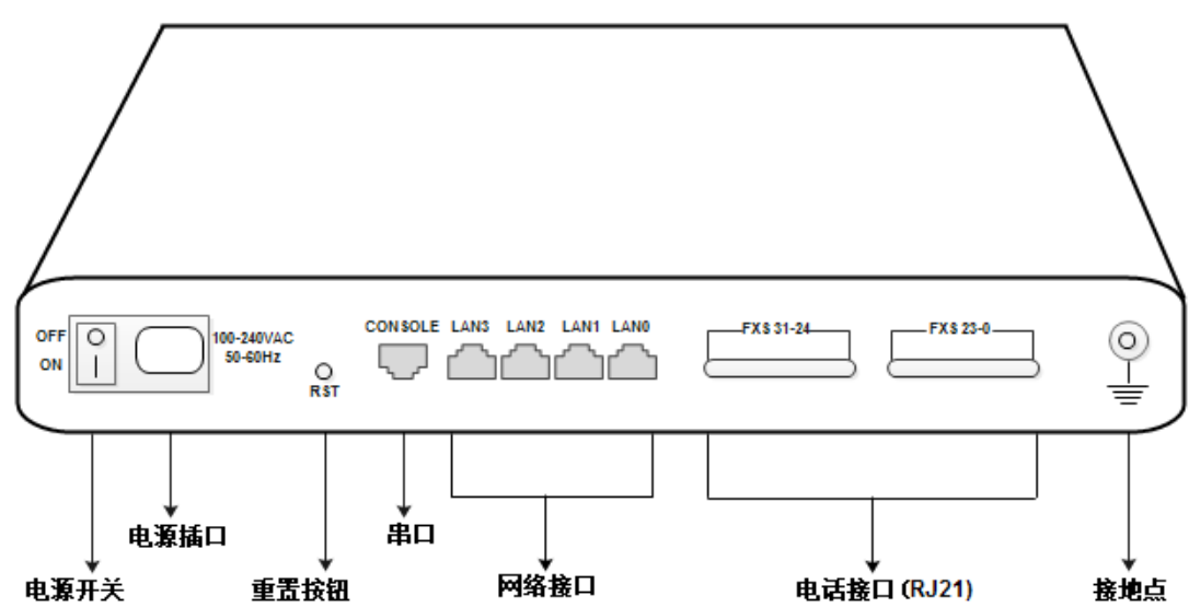
DAG2000-32S 接口和按钮说明
